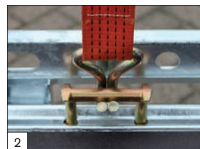
2 Standard: ganci fissaggio carico a scomparsa certificati TÜV con portata di 1000 kg per ogni punto.
